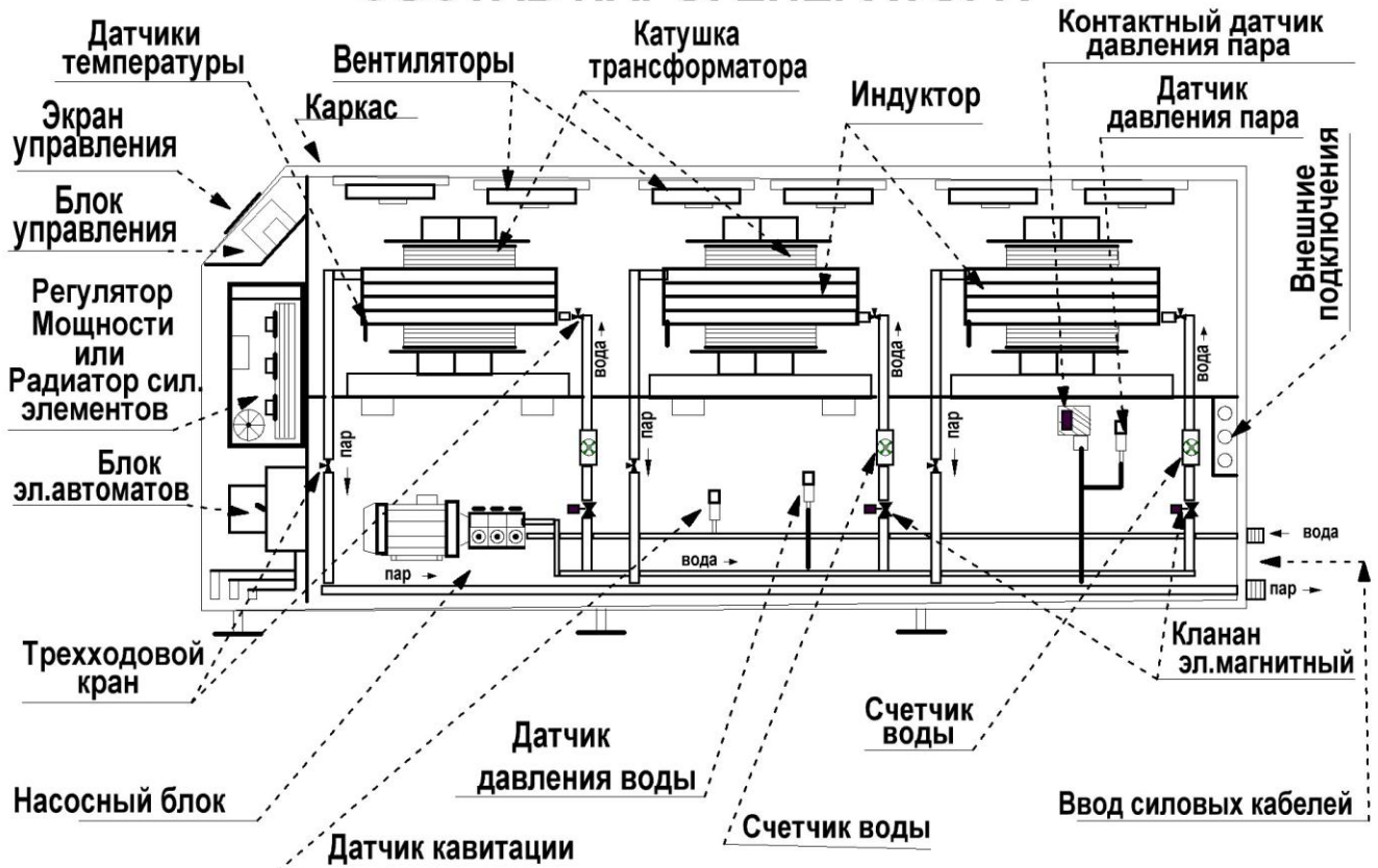
Рис. 3 Состав парогенератора с тремя индукторами.
