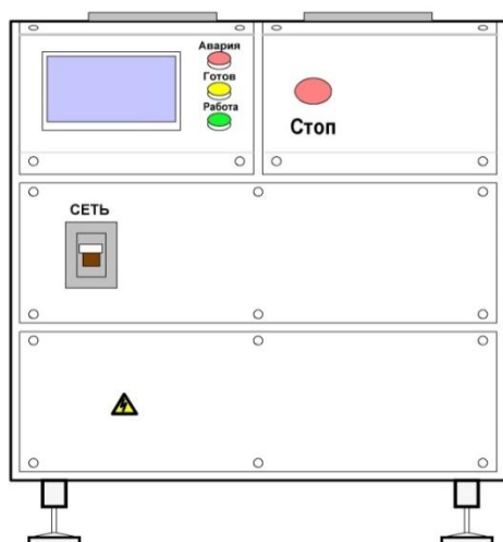
Вид спереди Парогенератора ТИТАН
